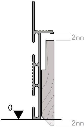
MONTAGGIO CON FUGA E BATTISCOPA TAGLIATO Installation with joint and cut skirting board Pose avec joint et plinthe découpée Montaje con fuga y rodapié cortado Montage mit Fuge und geteilter Sockelleiste Установка с обрезкой плинтуса и заделкой шва
