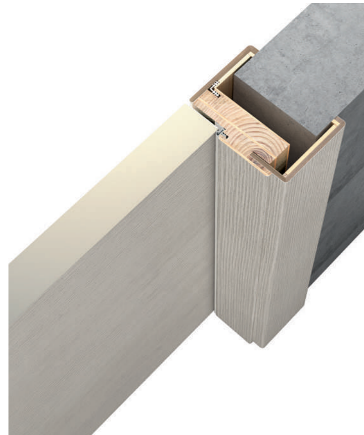
sezione No-Limits telaio standard standard section No-Limits frame section No-Limits cadre standard sección No-Limits bastidor estándar Querschnitt des No-Limits-Standardrahmens сечение двери No-Limits со стандартной рамой
