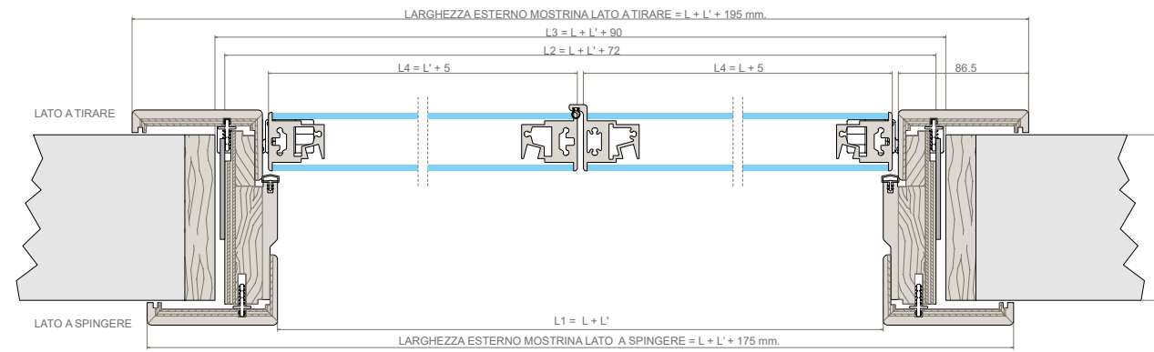
SEZIONE ORIZZONTALE
