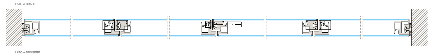
SEZIONE ORIZZONTALE
