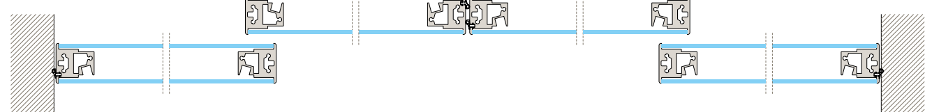
SEZIONE ORIZZONTALE
