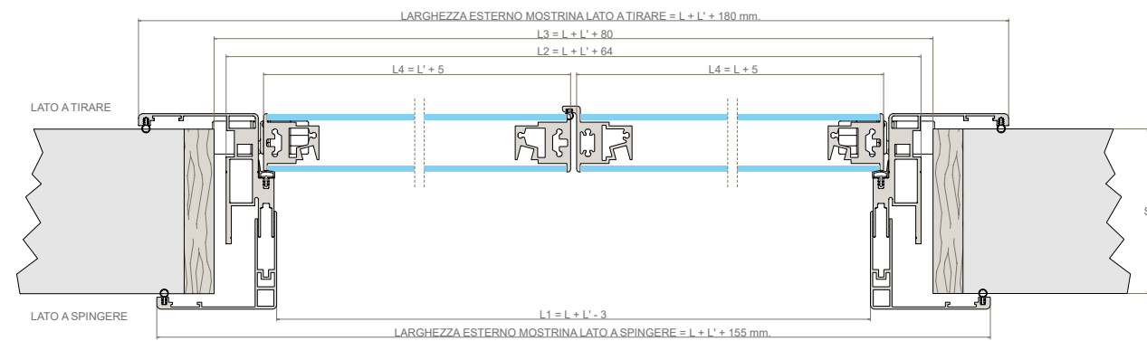
SEZIONE ORIZZONTALE
