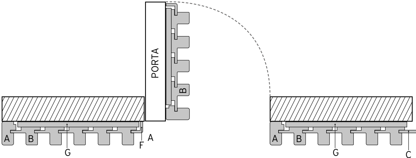
PARETE DRITTA CON PORTA | STRAIGHT WALL WITH DOOR | MUR DROIT AVEC PORTE | PARED RECTA CON PUERTA | GERADE WAND MIT TÜR | ПРЯМАЯ СТЕНА С ДВЕРЬЮ
