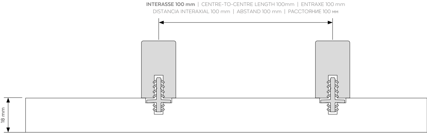
PANNELLO BOISERIE FISSATA A MURO | WALL-MOUNTED PANEL | PANNEAU BOISERIE FIXÉE AU MUR PANEL DE BOISERIE FIJADO EN PARED | AN DER WAND BEFESTIGTE TÄFELUNGSPLETTE | ПАНЕЛЬ, ПРИКРЕПЛЕННАЯ К СТЕНЕ
