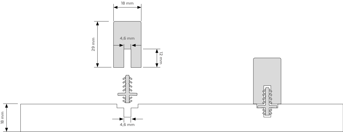
PANNELLO BOISERIE FISSATA A MURO | WALL-MOUNTED PANEL | PANNEAU BOISERIE FIXÉE AU MUR PANEL DE BOISERIE FIJADO EN PARED | AN DER WAND BEFESTIGTE TÄFELUNGSPLETTE | ПАНЕЛЬ, ПРИКРЕПЛЕННАЯ К СТЕНЕ
