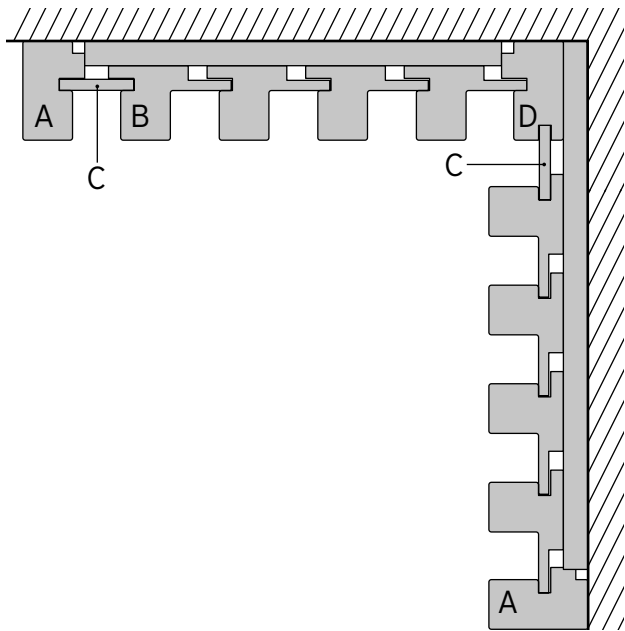
PARETE ANGOLO INTERNO | INTERIOR CORNER WALL | MUR D'ANGLE INTÉRIEUR | PARED ÁNGULO INTERNO | WAND MIT INNENWINKEL | ВНУТРЕННИЙ УГОЛ СТЕНЫ
